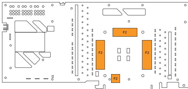
F2 Thermal Pad F 2 mm
