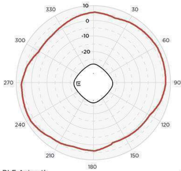
BLE Azimuth
