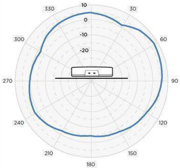
BLE Elevation
