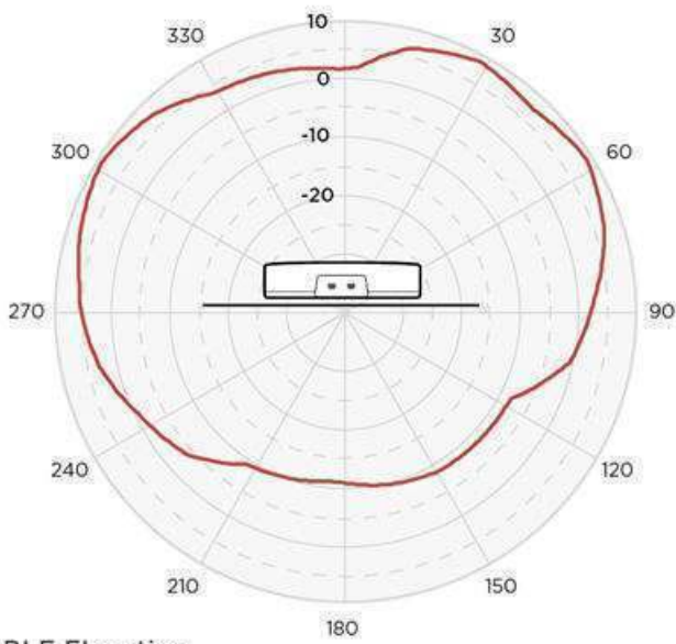
BLE Elevation
