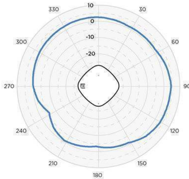
BLE Azimuth
