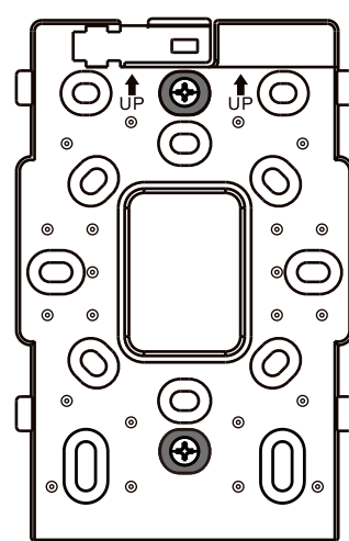
Распределительная коробка американского стандарта размером 108 мм x 59 мм
